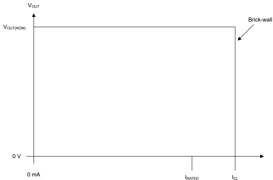
图 7-1. Current Limit
