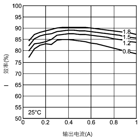
25°C · 输入5V时的效率
