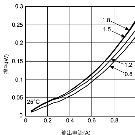
25°C · 输入4.5V时的消耗
