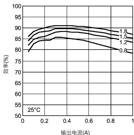
25°C · 输入4.5V时的效率
