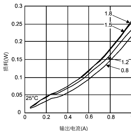
25°C · 输入5V时的消耗
