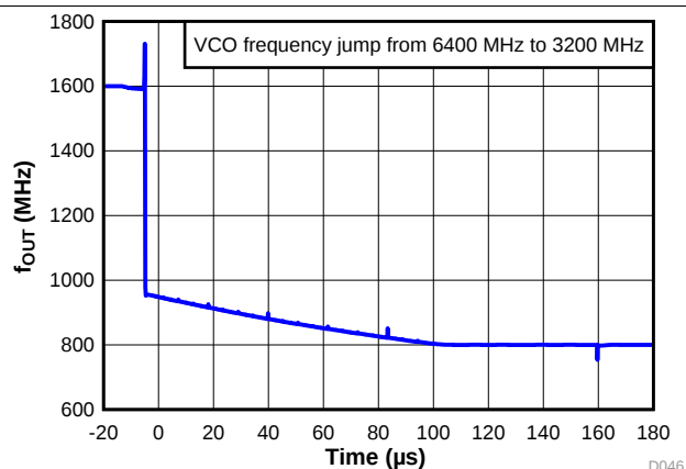
图 16. VCO Calibration Time
