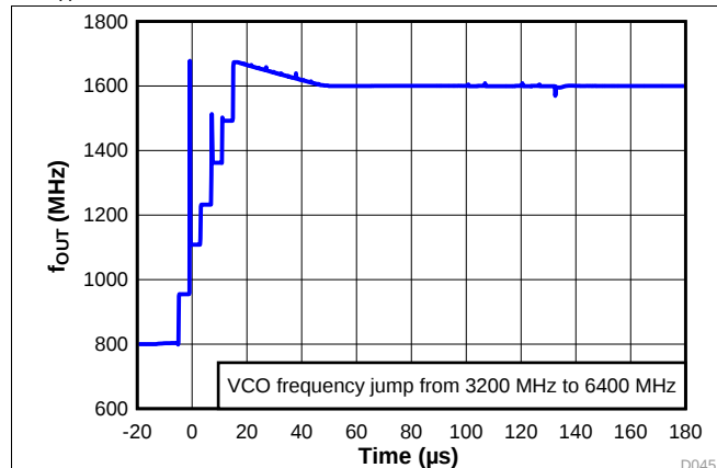
图 15. VCO Calibration Time
