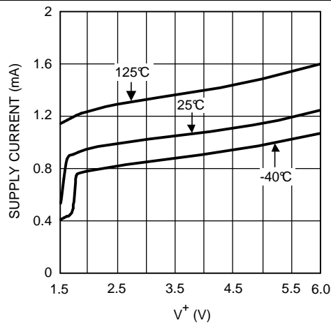
图 1. 电源电流与电源电压间的关系 (LMV791)
