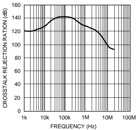
图 35. 串扰抑制
