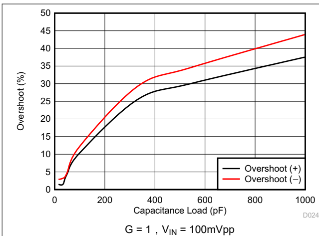
图 5-19. 小信号过冲与容性负载间的关系
