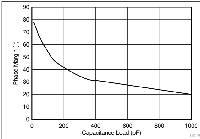
图 5-21. 相位裕度与容性负载间的关系
