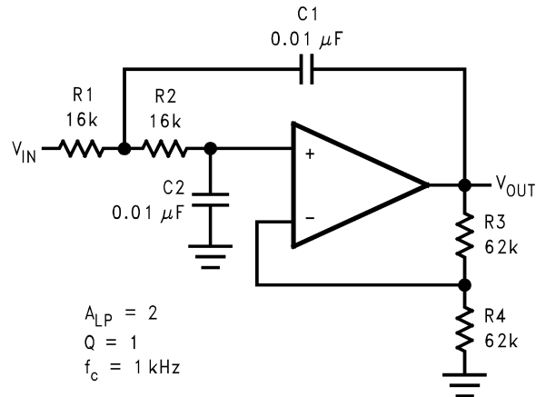
图 9-8. Sallen-Key 二阶有源低通滤波器
