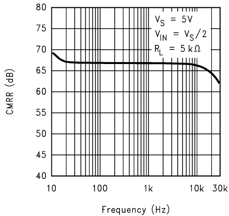
图 7-13. CMRR 与频率之间的关系
