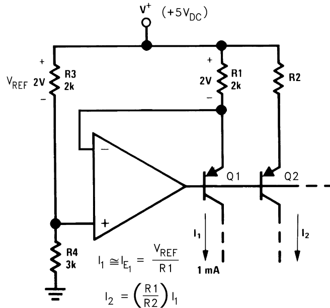
图 9-15. 固定拉电流
