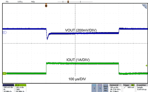
图 8-11. 负载瞬态
