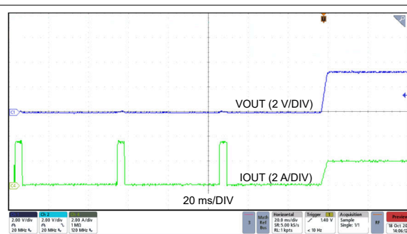
图 7-15. 退出断续
