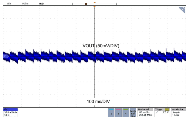
图 8-13. 负载瞬态
