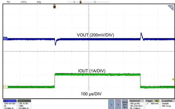
图 8-10. 负载瞬态
