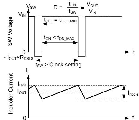
图 7-11. 压降波形
