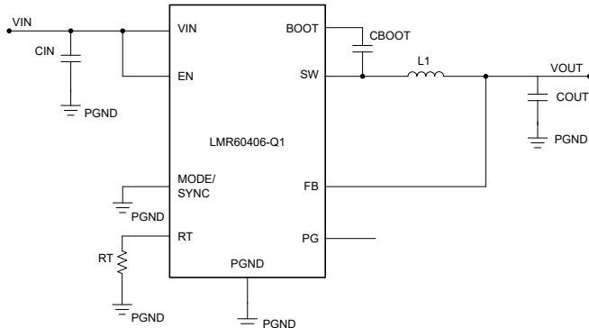
简化版原理图 - 固定输出
