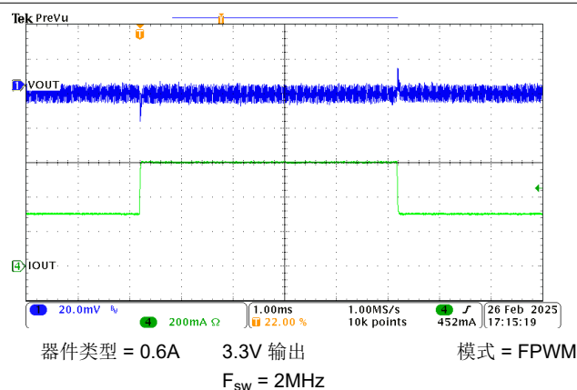
图 8-17. 0.3A 至 0.6A 负载瞬态
