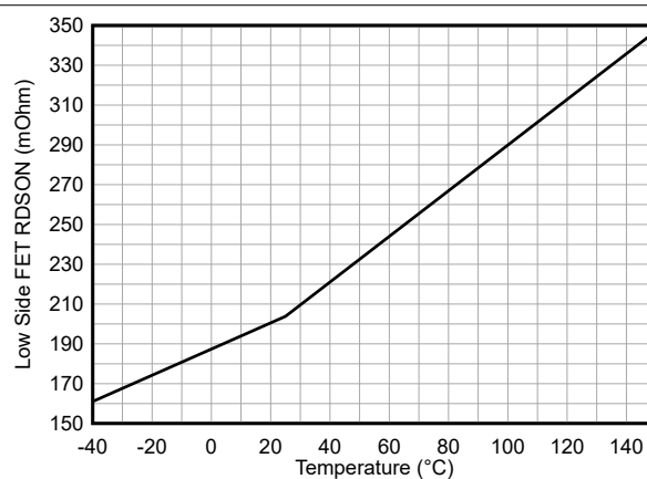
图 6-4. 低侧 MOSFET R_{DS-ON}
