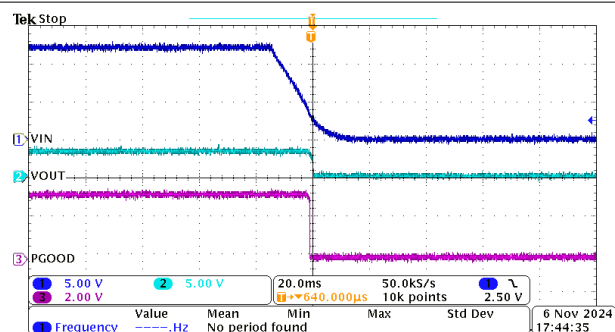
图 8-15. 关断
