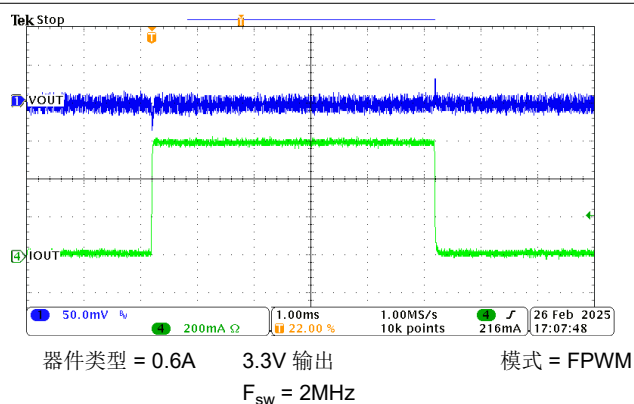
图 8-16. 0A 至 0.6A 负载瞬态
