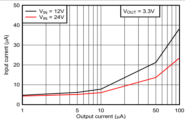
图 8-13. 轻负载条件下输入电流与负载电流间的关系
