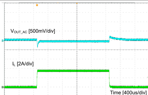
图 8-7. 负载瞬态
