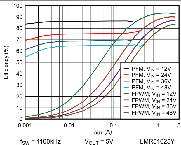
图 6-8. 效率与负载电流间的关系 (5V)
