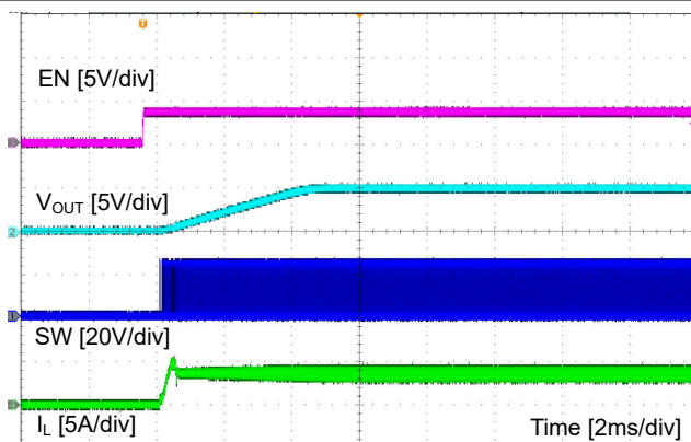
图 8-5. 由 EN 启动
