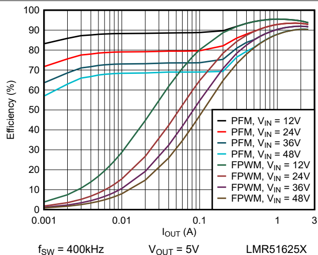
图 6-6. 效率与负载电流间的关系 (5V)
