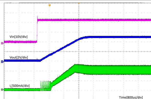
图 8-5. 由 V_{IN} 启动
