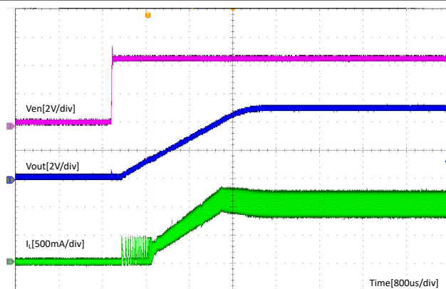
图 8-6. 由 EN 启动
