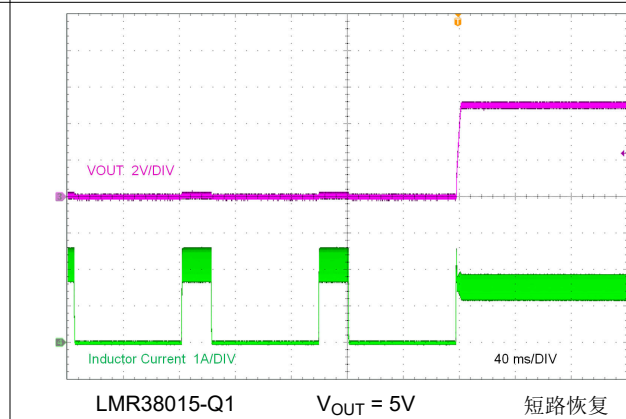
图 8-8. 短路恢复
