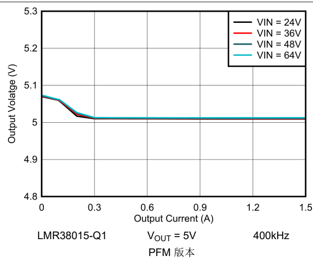
图 8-13. 5V 负载调节
