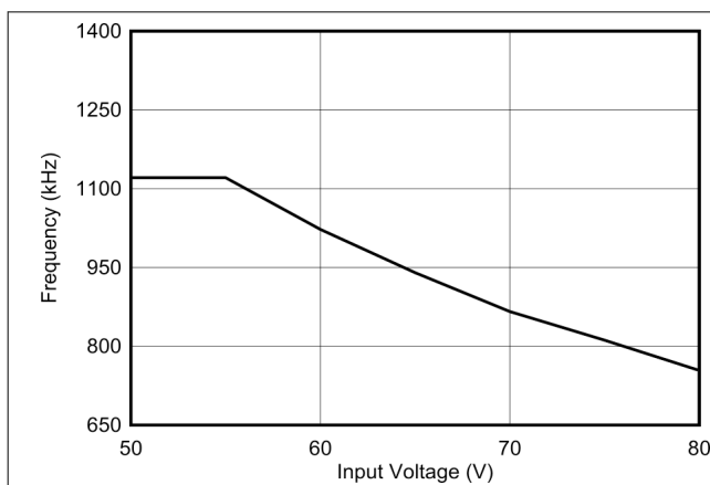
图 7-7. T_{ON\_MIN} 时的典型频率折返
