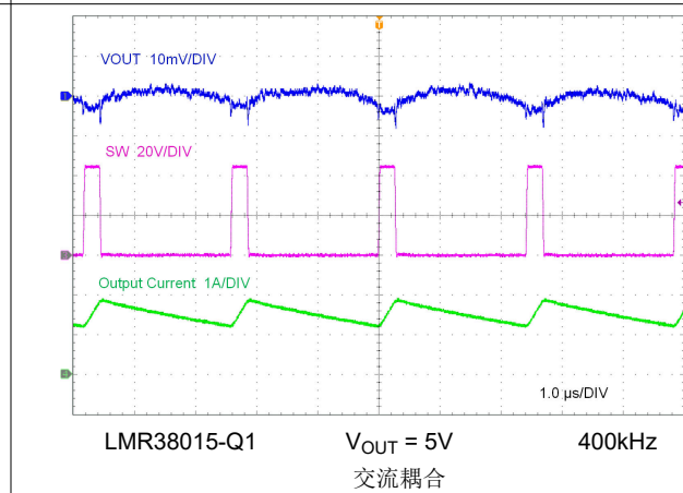
图 8-6. 满载开关
