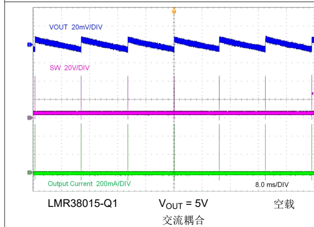
图 8-5. PFM 开关
