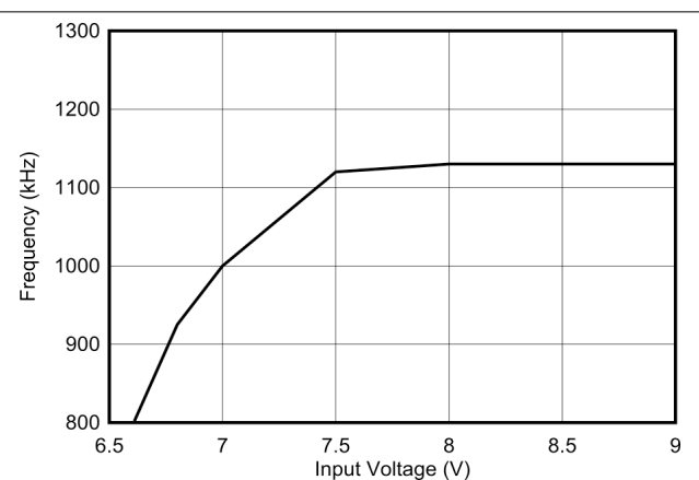
图 7-8. T_{OFF\_MIN} 时的典型频率折返
