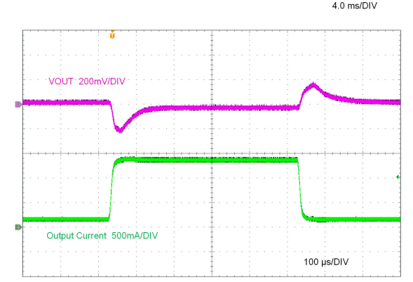
LMR38015-Q1 V_{OUT} = 5V 400kHz (交流耦合) 200mA/μs 时为 150mA 至 1350mA
