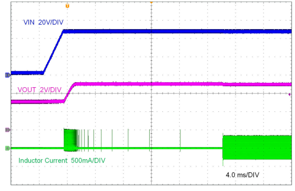
LMR38015-Q1 V_{OUT} = 5V 空载 偏置为 3V
