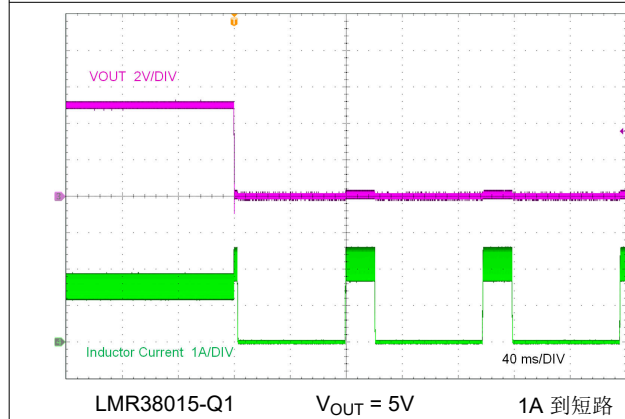
图 8-7. 应用短路
