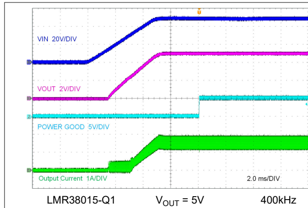
图 8-3. 由 VIN 启动
