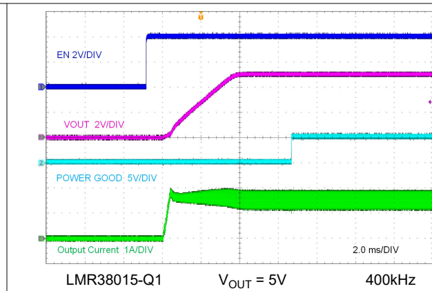
图 8-4. 由 EN 启动
