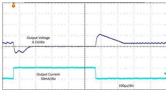
LMR36500P3 V_{OUT} = 3.3V (固定值) 1MHz (自动值)
