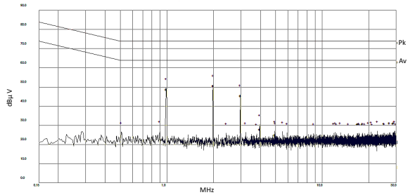
LMR36500P5 V_{OUT} = 5V (固定值) V_{IN} = 24V 无 EMI 滤波器 C_{IN} = 3x 2.2µF
