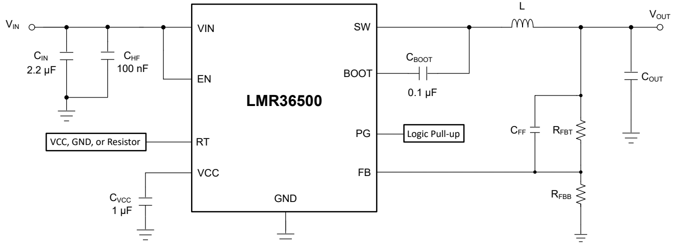
图 8-1. 应用电路示例：ADJ 输出电压模式
