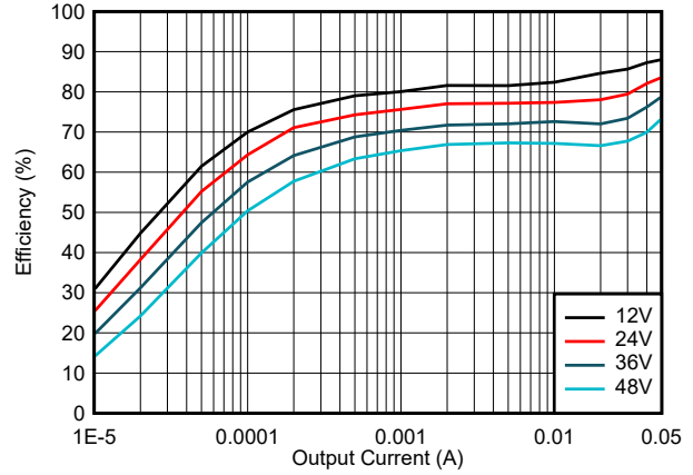
LMR36500P5 V_{OUT} = 5V (固定值) 600kHz (自动值)
