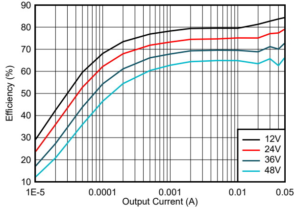
LMR36500P3 V_{OUT} = 3.3V (固定值) 600kHz (自动值)
