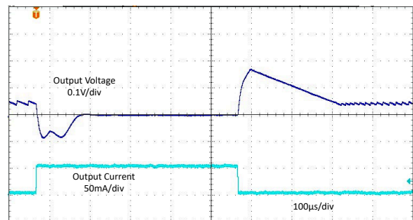
LMR36500P5 V_{OUT} = 5V (固定值) 1MHz (自动值)
