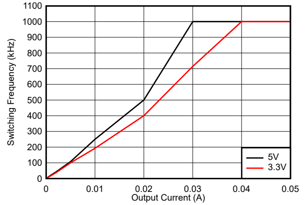
LMR36500P3 V_{IN} = 12V (固定值) 1MHz (自动值)
