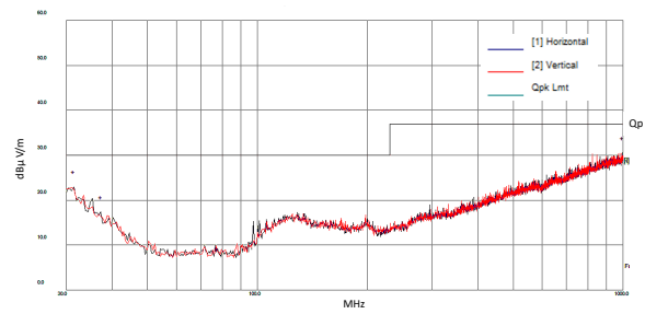
LMR36500P5 V_{OUT} = 5V (固定值) V_{IN} = 24V 无 EMI 滤波器 C_{IN} = 3x 2.2µF
