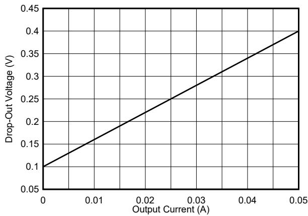
LMR36500P5 V_{OUT} = 5V (固定值) 1MHz (自动值)
