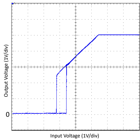
图 6-2. 输入电压 UVLO 阈值
