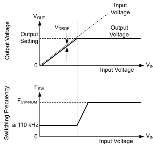
图 7-18. 压降中的频率和输出电压
