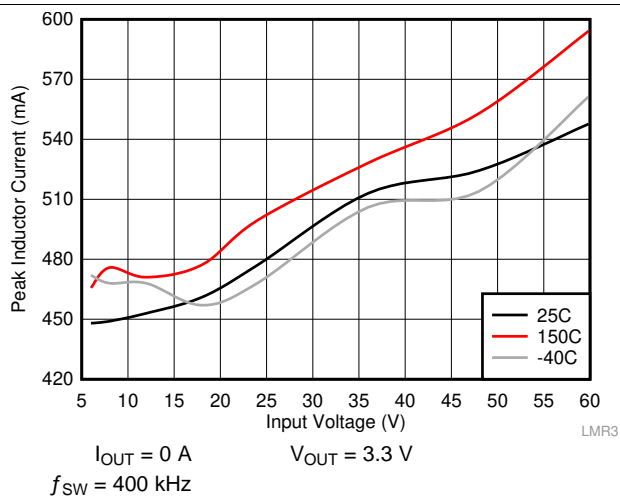
图 6. I_{PEAK-MIN}
