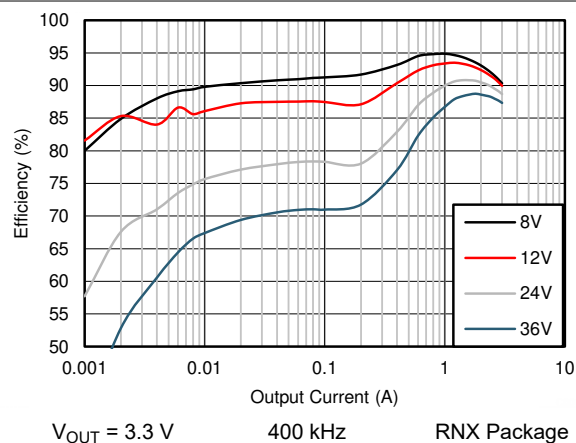
图 9-6. Efficiency
