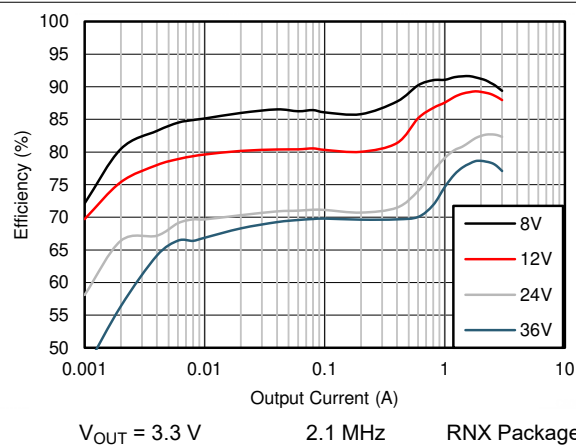
图 9-8. Efficiency
