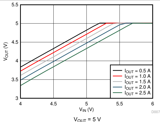
图 6-7. Dropout Curve
