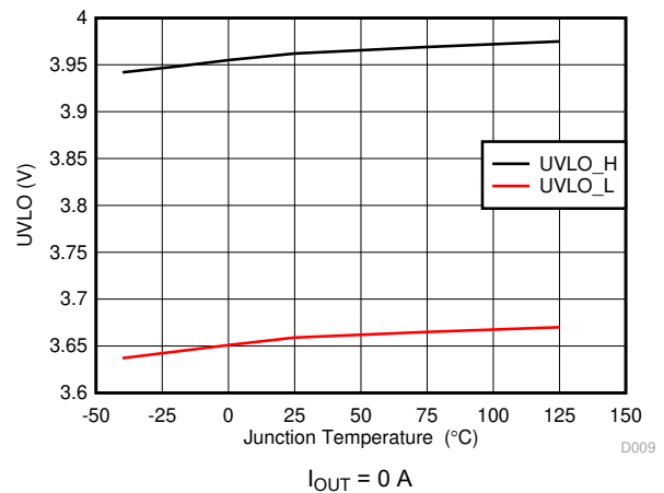
图 6-12. UVLO Threshold
