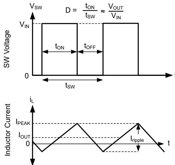
图 8-16. FPWM Mode Operation
