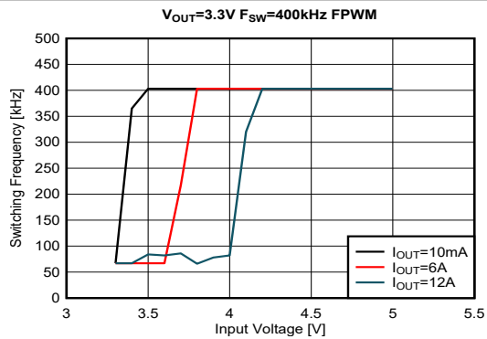
图 9-33. Dropout
