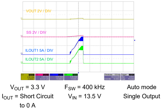
图 9-43. Short-Circuit Hiccup
