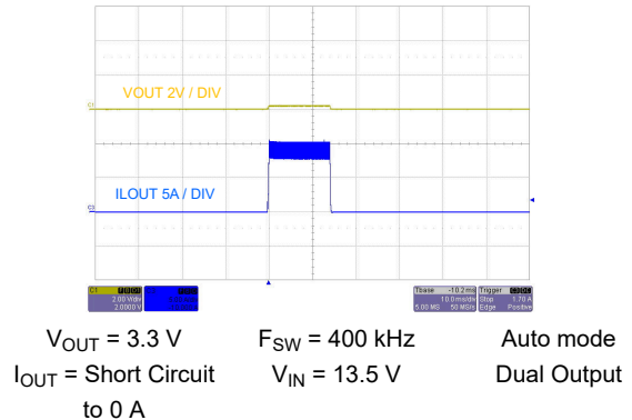
图 9-44. Short-Circuit Hiccup
