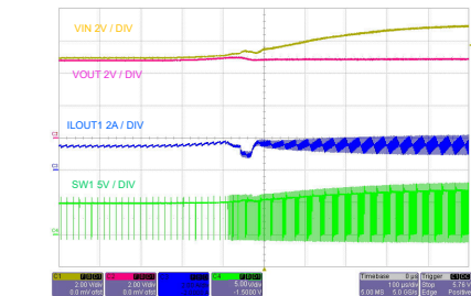
图 9-35. Dropout
