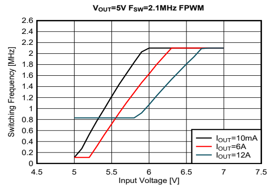
图 9-34. Dropout
