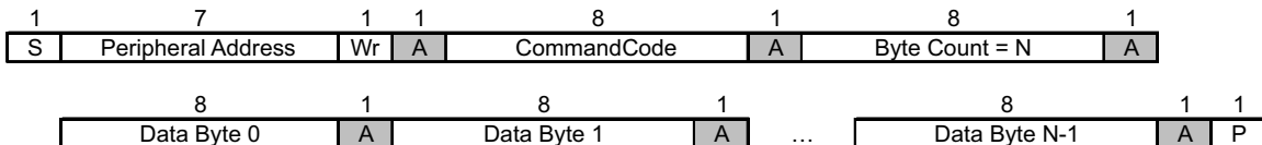
图 8-10. 块写入协议
