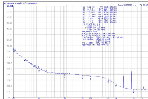
图 6-19. 100 MHz Output Phase Noise (APLL1)
