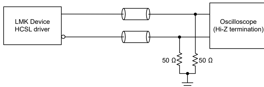
图 7-7. HCSL Output Time Domain Test Configuration
