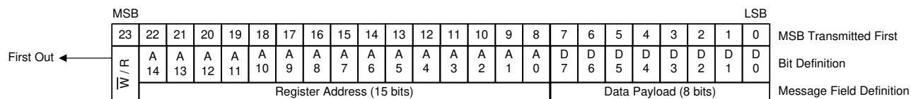
图 8-43. SPI Message Format
