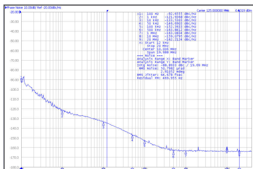
图 6-10. 125-MHz Output Phase Noise (APLL3 BAW)
