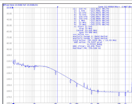
图 6-8. 312.5 MHz Output Phase Noise (APLL3 BAW)
