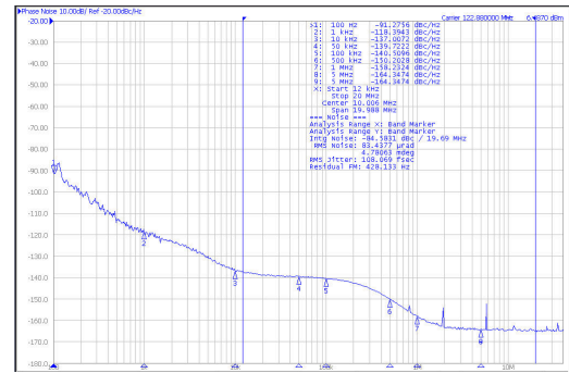
图 6-17. 122.88 MHz Output Phase Noise (APLL2)
