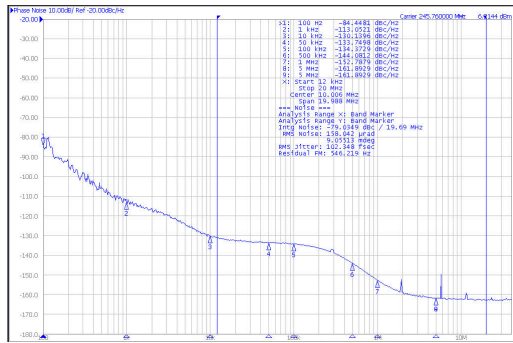
图 6-16. 245.76-MHz Output Phase Noise (APLL2)
