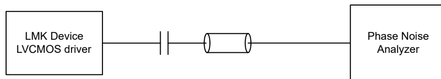
图 7-4. LVC MOS Output Phase Domain Test Configuration
