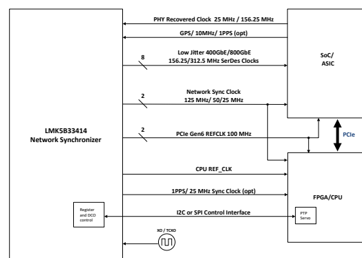
LMK5B33414 典型系统方框图
