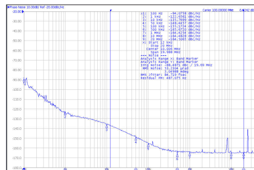
图 6-11. 100 MHz Output Phase Noise (APLL3 BAW)
