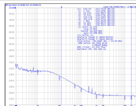
图 6-9. 156.25-MHz Output Phase Noise (APLL3 BAW)
