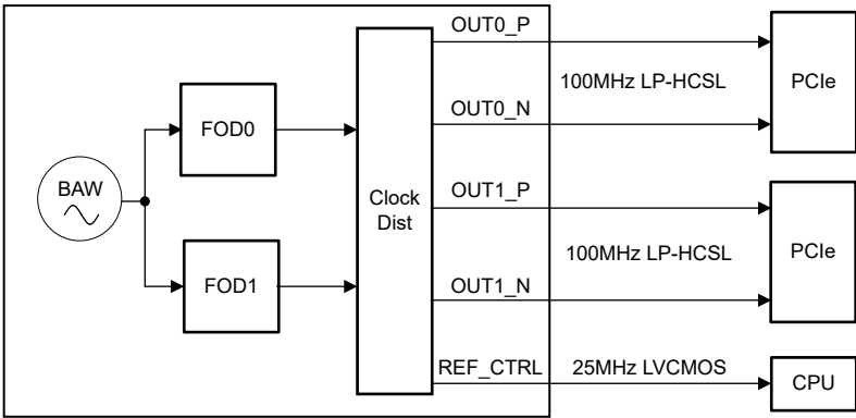
图 9-1. PCIe 应用
