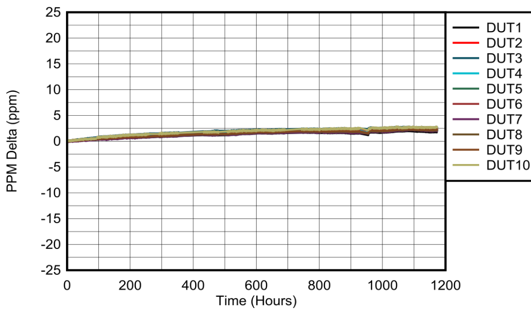
图 9-9. 频率随时间变化的稳定性 — 3.3V 电源电压
