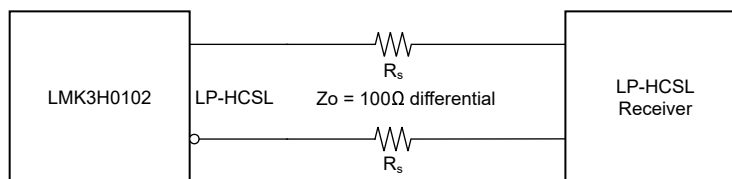
图 7-8. 将 LMK3H0102-Q1 LVCMOS 输出与 LP-HCSL 接收器相连接
