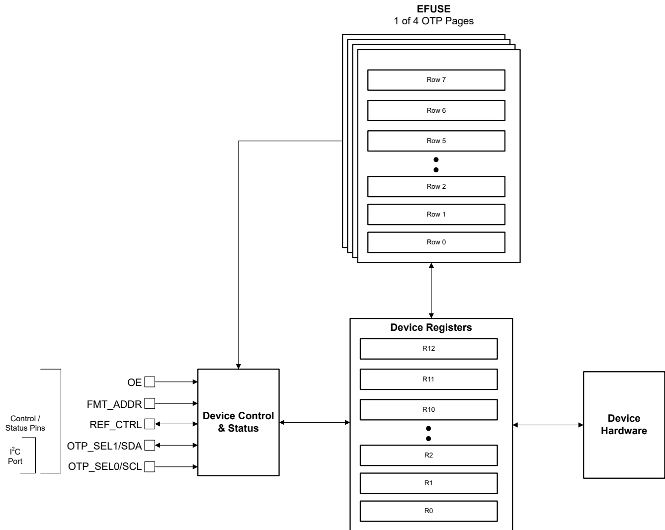
图 7-3. LMK3H0102-Q1 接口和控制块
