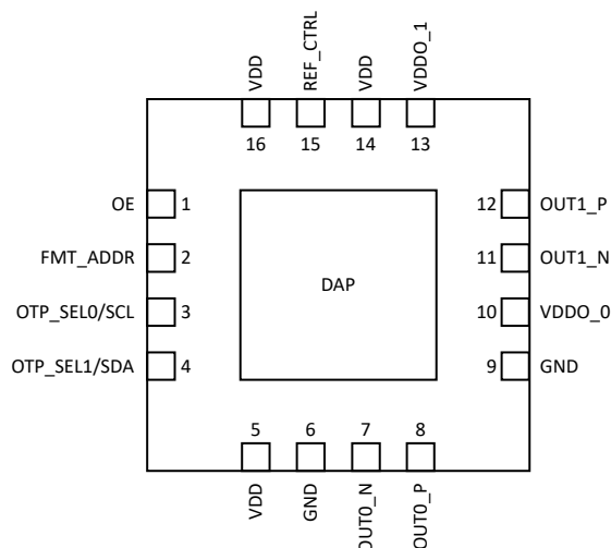
图 4-1. LMK3H0102-Q1 16 引脚 VQFN 顶视图
