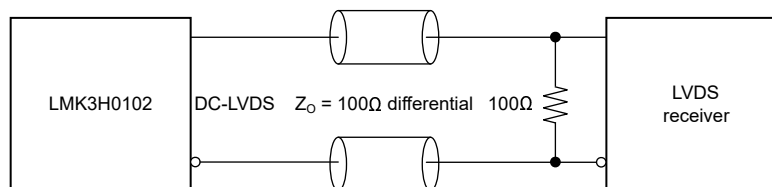
图 7-7. 将 LMK3H0102-Q1 LVCMOS 输出与直流 LVDS 接收器相连接
