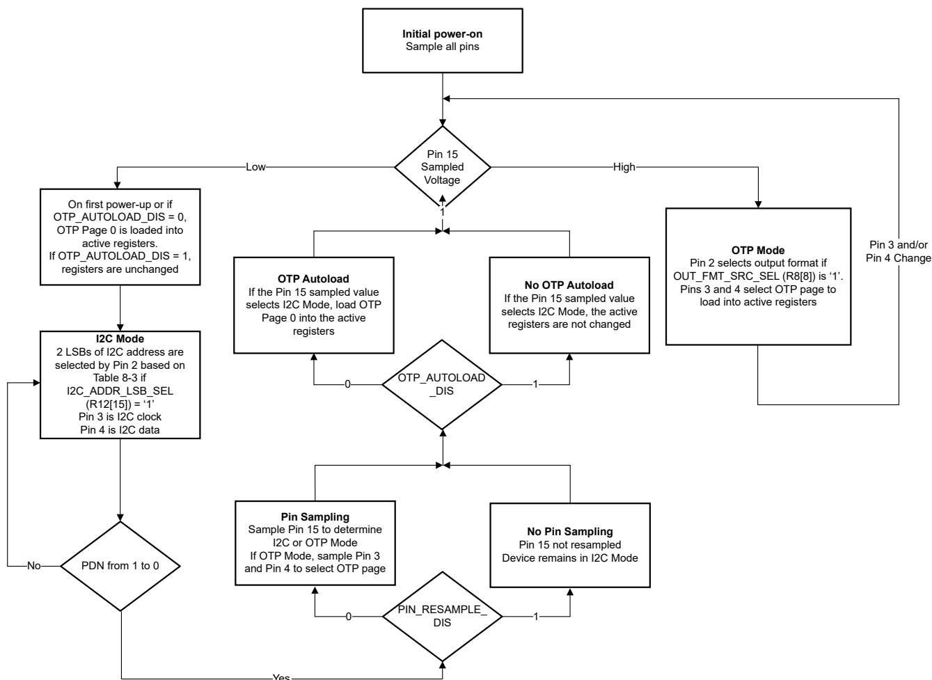
图 7-2. LMK3H0102-Q1 器件模式图
