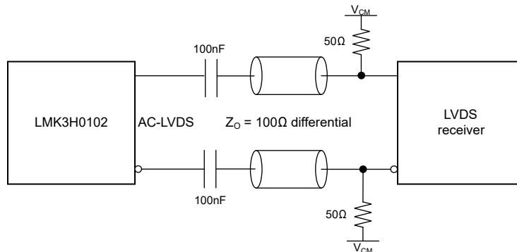
图 7-6. 将 LMK3H0102-Q1 LVCMOS 输出与交流 LVDS 接收器相连接
