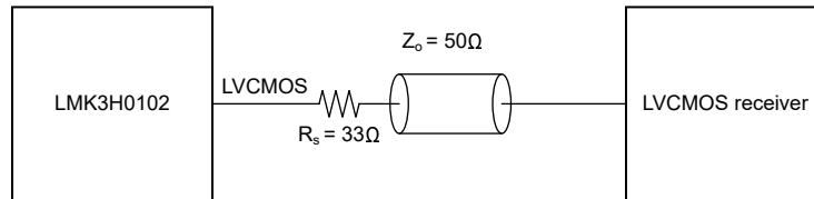
图 7-5. 将 LMK3H0102-Q1 LVCMOS 输出与 LVCMOS 接收器相连接
