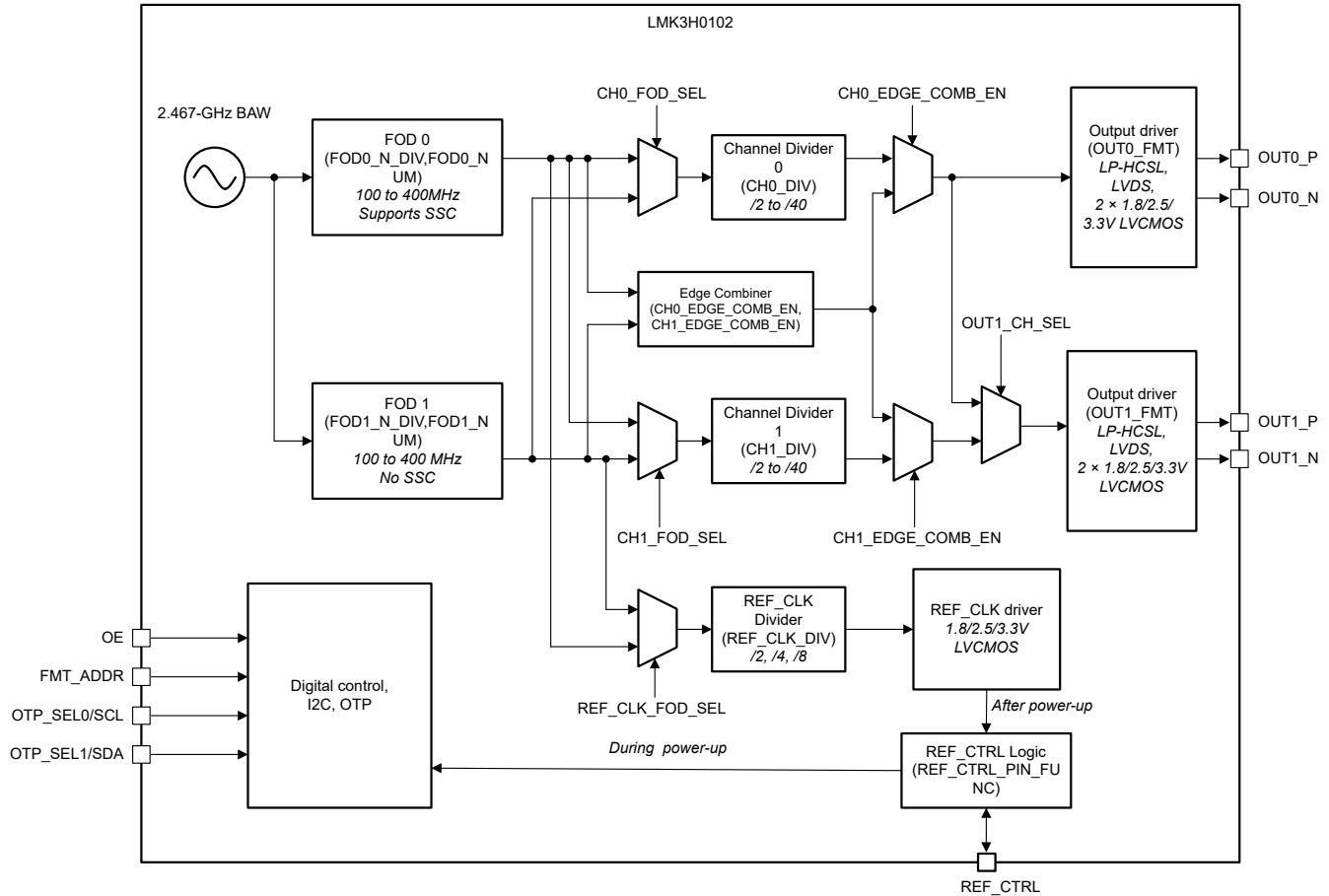
图 7-1. LMK3H0102-Q1 功能方框图
