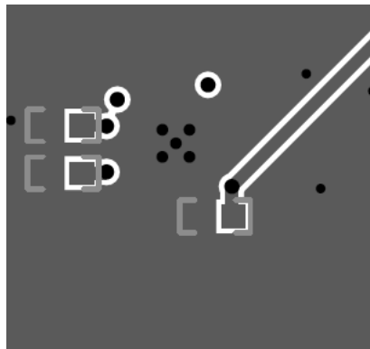
图 9-12. LMK3H0102-Q1 的 PCB 布局示例，底层
