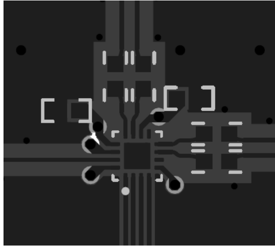
图 9-11. LMK3H0102-Q1 的 PCB 布局示例，顶层
