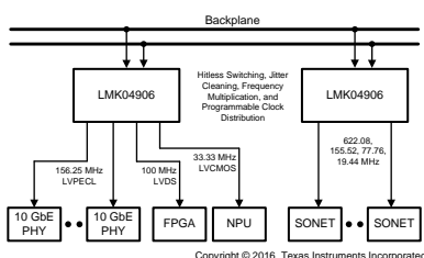
系统应用图
