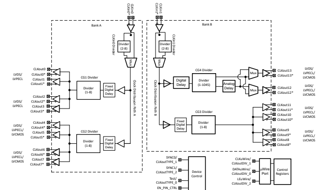
功能方框图
