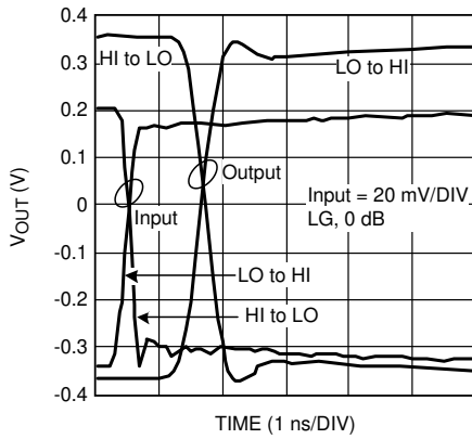
图 5-37. Step Response
