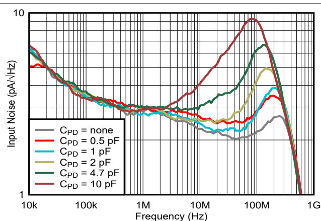
图 7-4. Input Noise Density vs Input Capacitance
