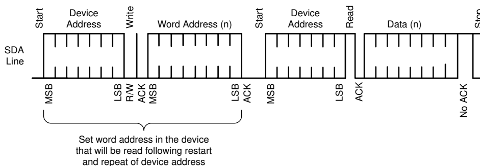
图 8-7. SMBus Read Operation
