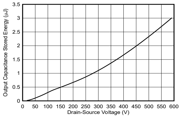
图 5-3. 输出电容储存能量与漏源电压之间的关系
