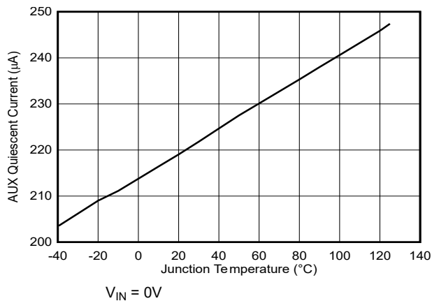
图 5-5. AUX 静态电流与结温间的关系
