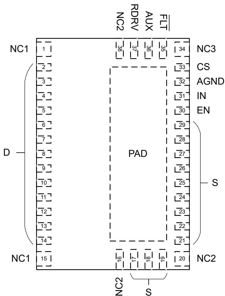
图 4-1. REQ 封装，38 引脚 VQFN (俯视图)
