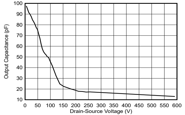
图 5-2. 输出电容与漏源电压之间的关系
