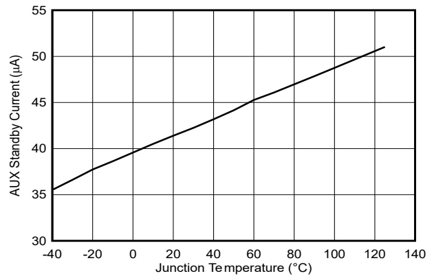
图 5-4. AUX 待机电流与结温间的关系
