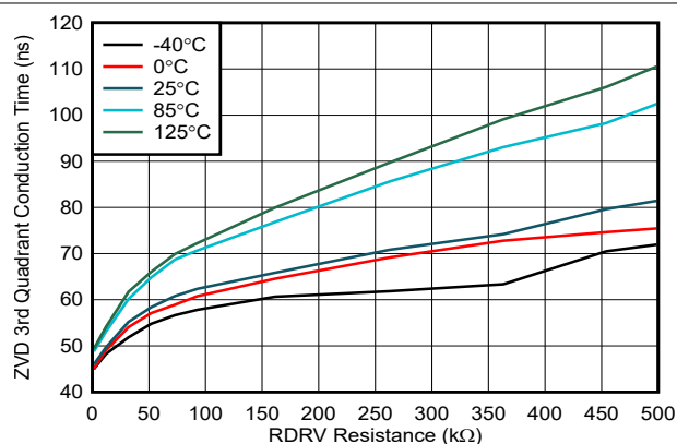
图 5-12. ZVD 第三象限导通时间与驱动强度电阻之间的关系
