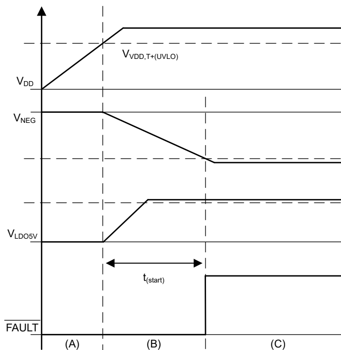
图 7-10. 启动时序图
