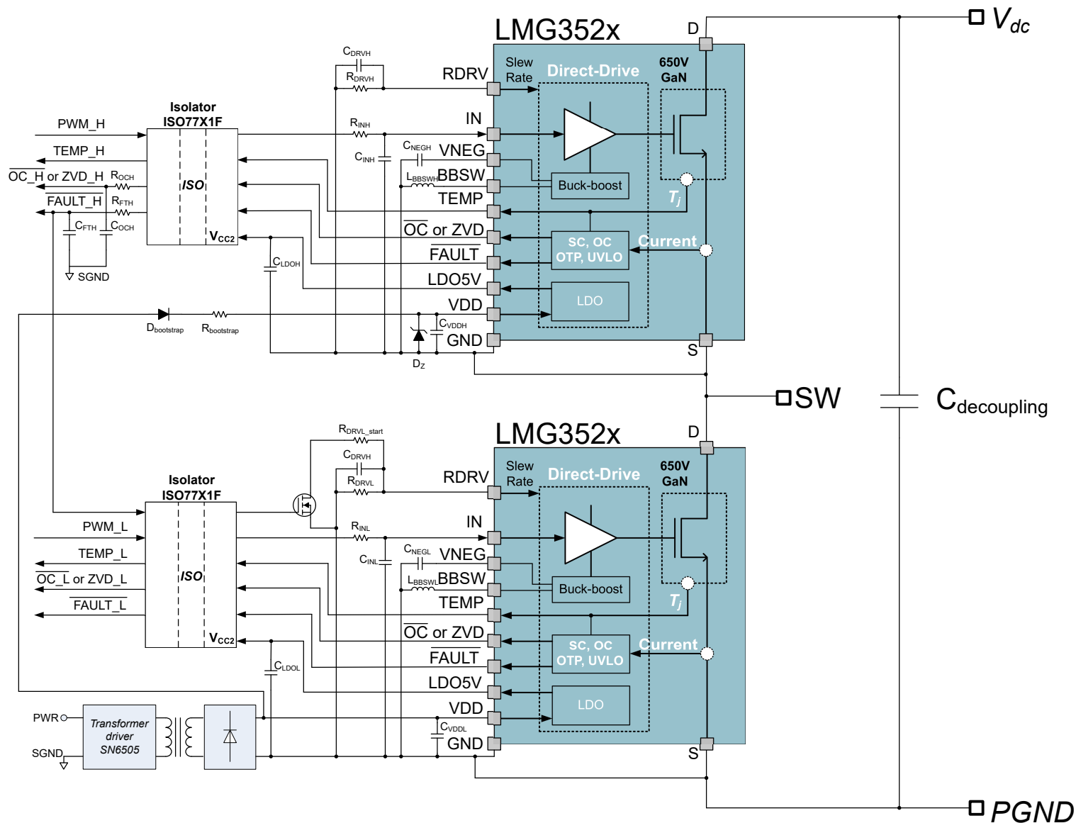
图 8-2. 具有自举功能的典型半桥应用
