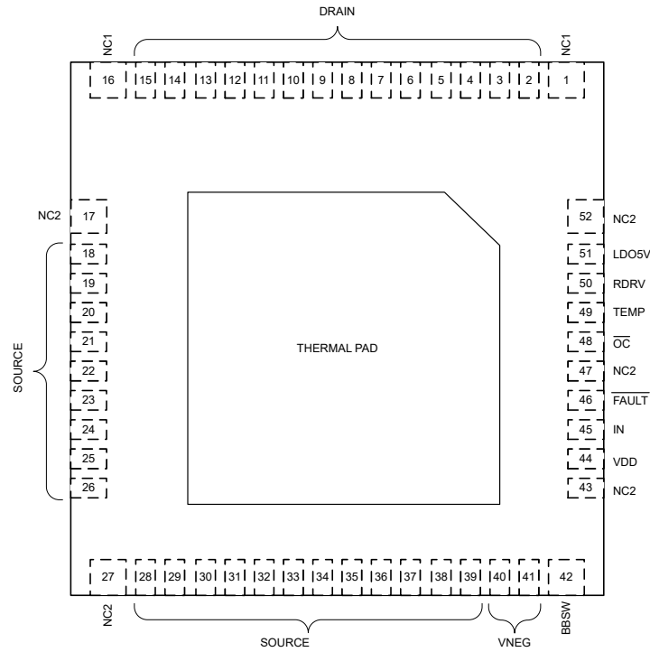
图 4-1. LMG3522R050 RQS 封装 52 引脚 VQFN (顶视图)
