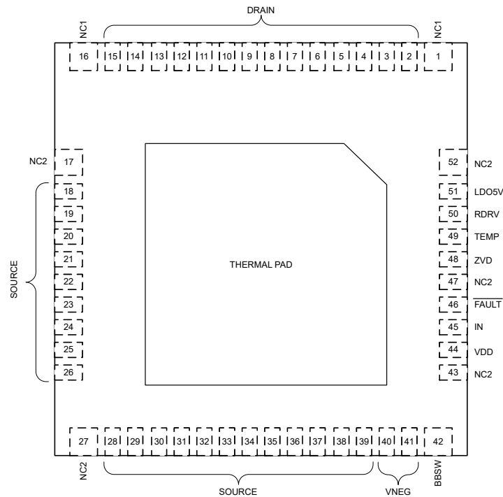
图 4-2. LMG3526R050 RQS 封装 52 引脚 VQFN (顶视图)
