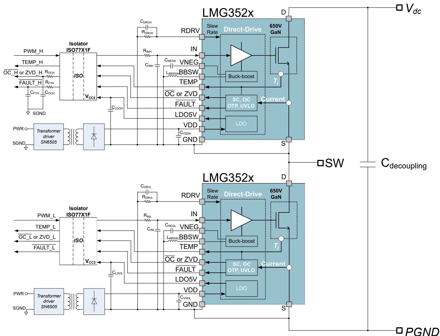
图 8-1. 采用隔离式电源的典型半桥应用
