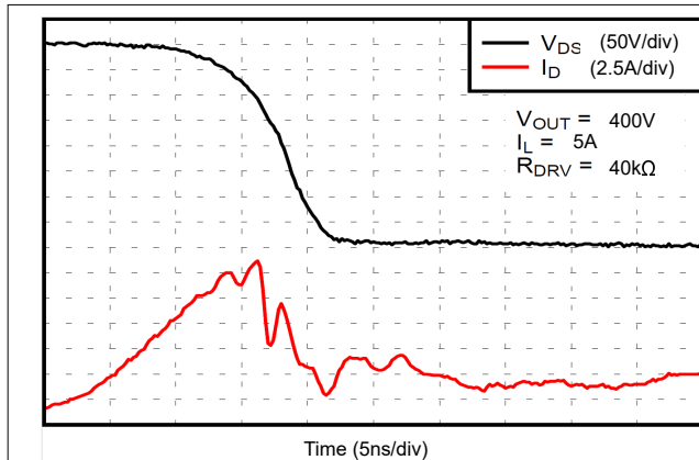
图 8-5. 应用示例中的导通波形
