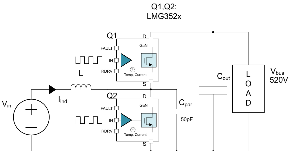
图 6-4. 安全工作区曲线所用电路
