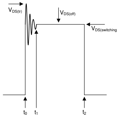
图 7-1. 漏源电压开关周期
