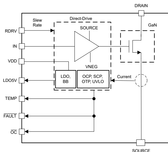
簡化版方框图
