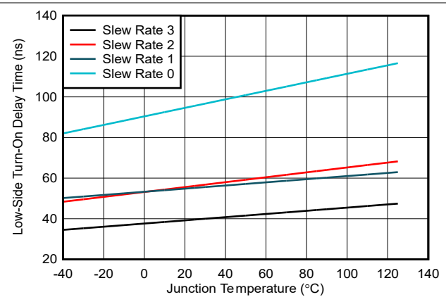
图 5-6. 低侧导通延迟时间与结温间的关系
