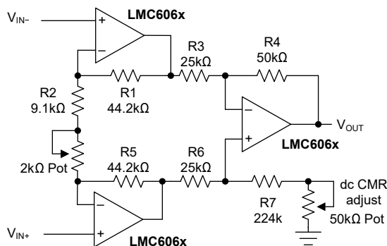
图 6-4. 仪表放大器
