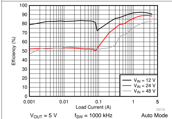
图 27. LM76003 Efficiency
