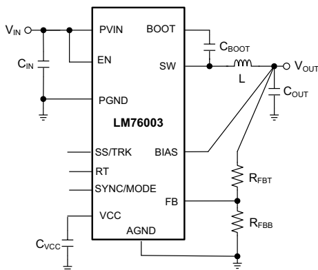
简化原理图
