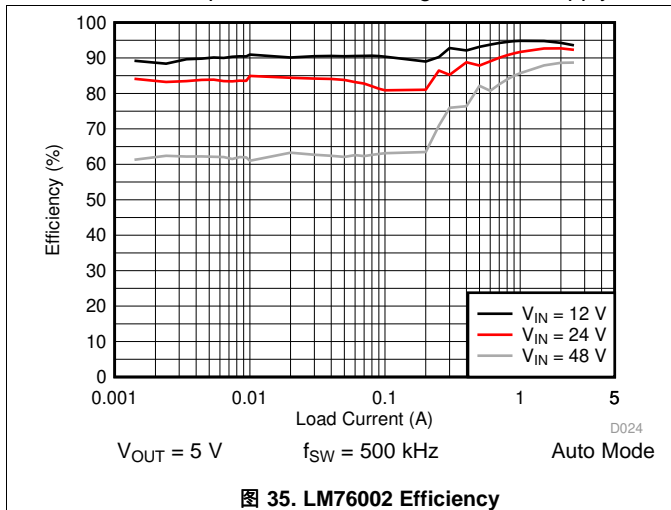
图 35. LM76002 Efficiency
