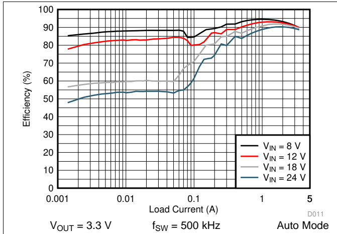
图 23. LM76003 Efficiency
