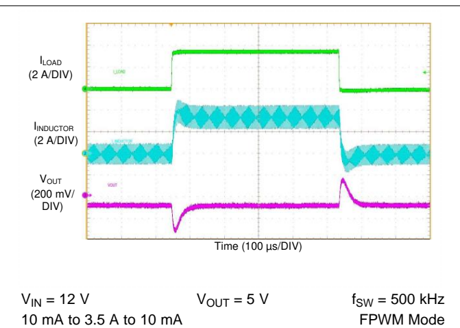
图 76. LM76003 Load Transient
