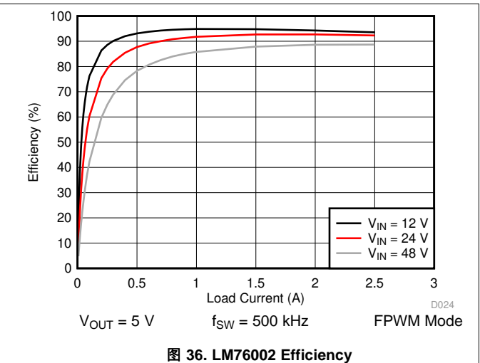
图 36. LM76002 Efficiency
