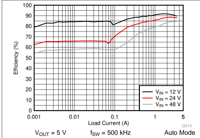
图 25. LM76003 Efficiency
