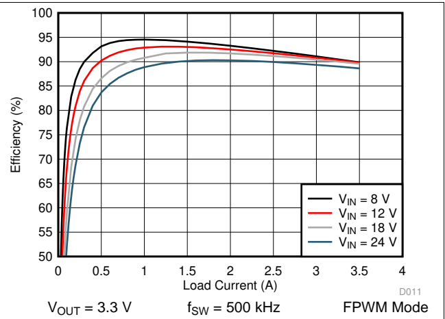
图 24. LM76003 Efficiency
