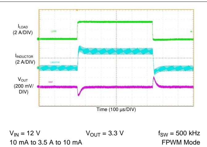
图 74. LM76003 Load Transient
