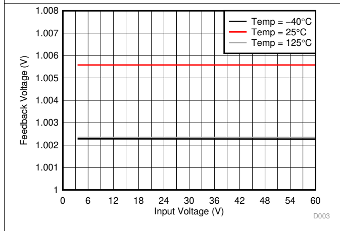
图 3. Feedback Voltage
