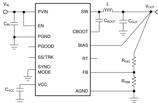
图 9-1. LM73605-Q1/6-Q1 Basic Schematic
