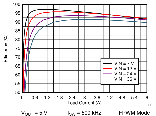
图 9-14. LM73606-Q1 Efficiency
