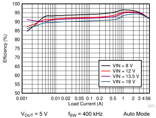
图 9-11. LM73606-Q1 Efficiency
