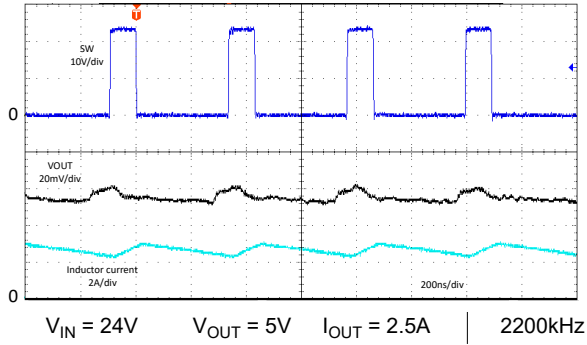
图 8-61. 典型开关波形 - LM6x625 - FPWM
