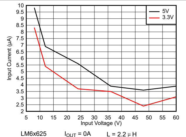
图 8-48. 空载输入电源电流 - 自动模式
