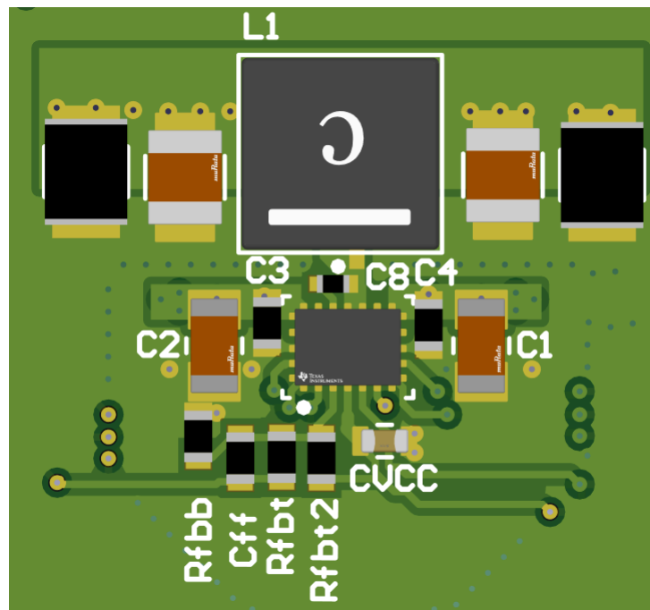
图 8-79. PCB 图像
