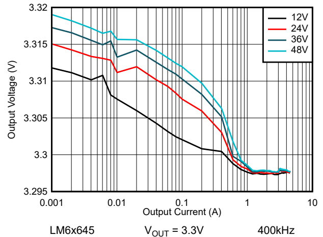
图 8-28. LM6x645 线路和负载调节 - 自动模式
