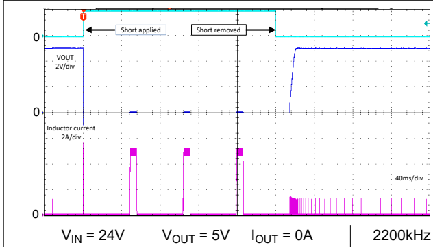
图 8-69. 输出短路电路和恢复 - 自动
