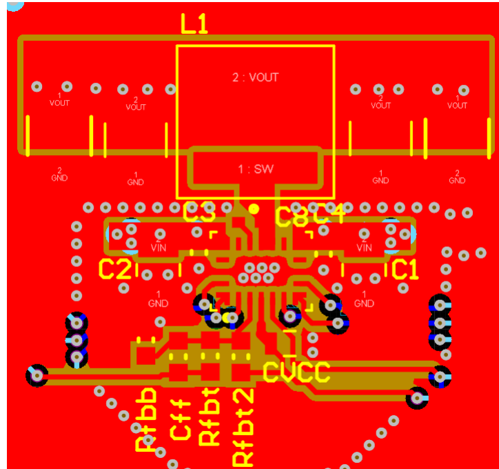
图 8-78. 布局示例
