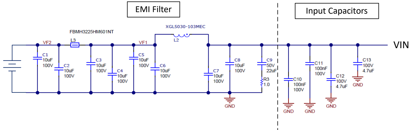
图 8-76. 适用于 400kHz 的 EMI 输入滤波器
