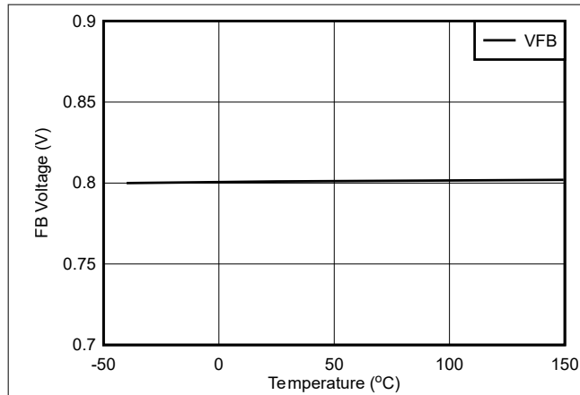
图 6-1. 反馈电压
