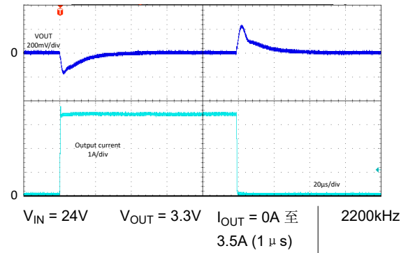
图 8-64. 负载瞬态 - LM6x635 - FPWM
