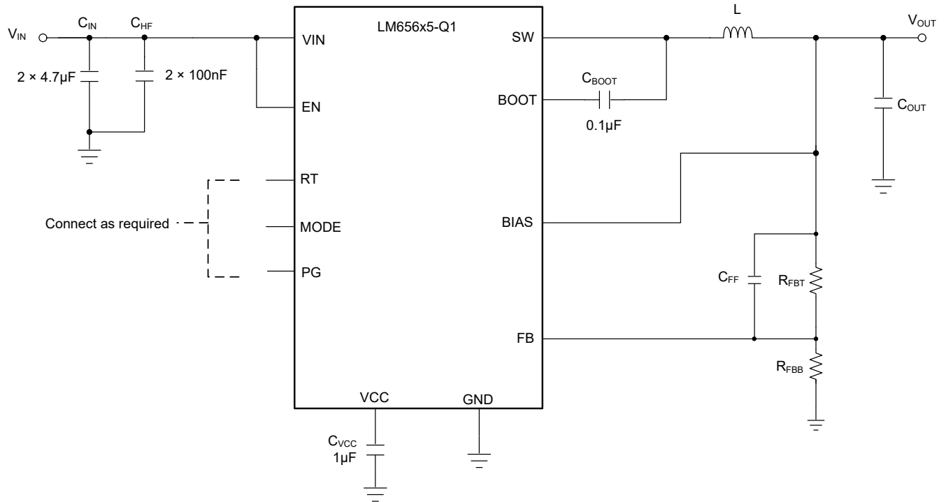
图 8-1. LM656x5-Q1 可调输出电压模式下的示例应用电路
