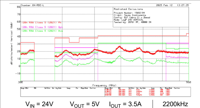
图 8-56. LM6x635 辐射 EMI - 对数周期 - 垂直
