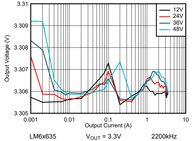
图 8-26. LM6x635 线路和负载调节 - 自动模式
