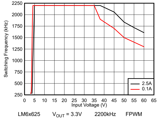
图 8-34. LM6x625 开关频率与输入电压间的关系
