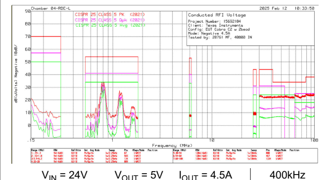
图 8-58. LM6x645 传导 EMI - 负向线路
