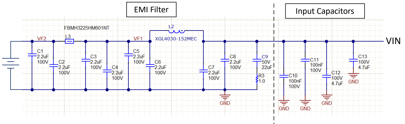
图 8-75. 适用于 2200kHz 的 EMI 输入滤波器
