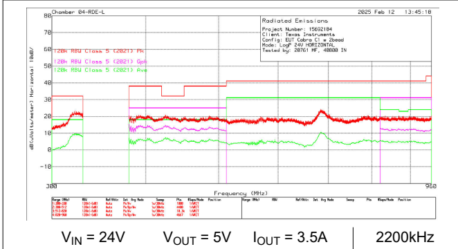
图 8-55. LM6x635 辐射 EMI - 对数周期 - 水平
