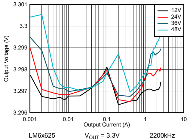
图 8-22. LM6x625 线路和负载调节 - 自动模式
