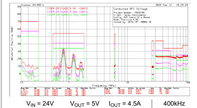
图 8-57. LM6x645 传导 EMI - 正向线路
