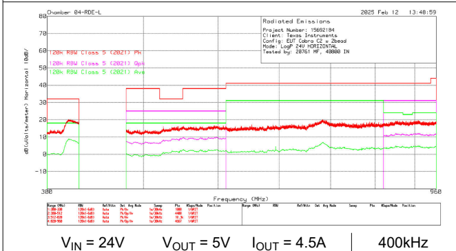
图 8-59. LM6x645 辐射 EMI - 对数周期 - 水平
