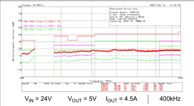
图 8-60. LM6x645 辐射 EMI - 对数周期 - 垂直
