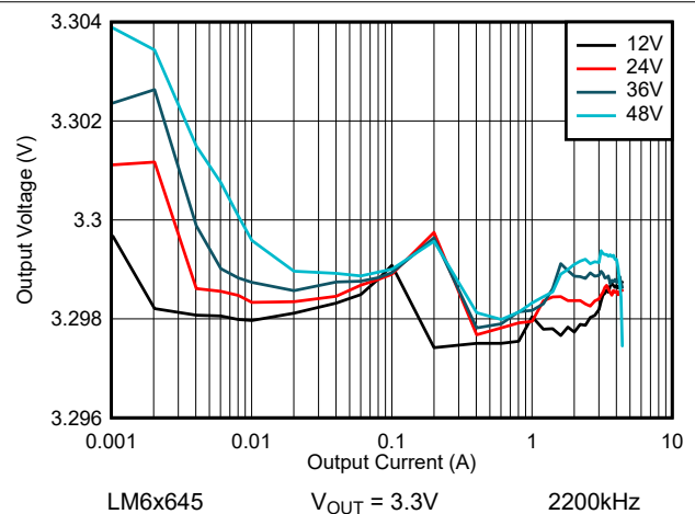
图 8-30. LM6x645 线路和负载调节 - 自动模式
