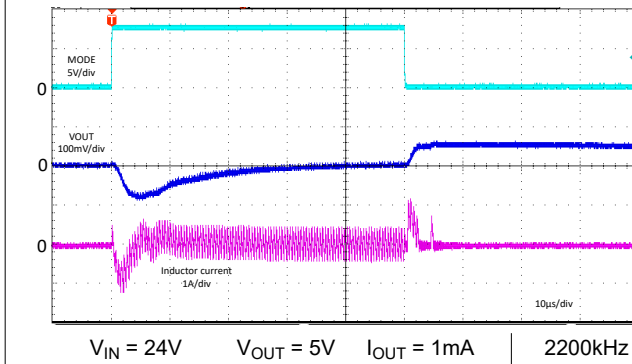
图 8-71. 模式变化瞬态
