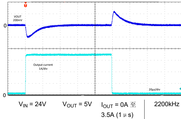
图 8-63. 负载瞬态 - LM6x635 - FPWM
