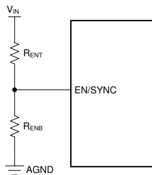
图 9-1. V_{IN} UVLO Using the EN pin
