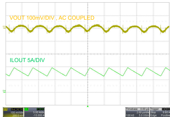
图 7-9. 输出纹波， V_{SUPPLY} = 48V ， I_{LOAD} = 8A
