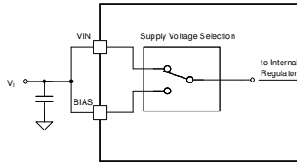
图 8-10. VMAX Supply Scenario 2
