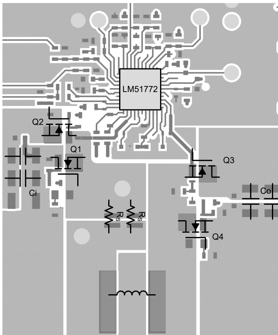
图 10-8. LM51772 Simplified Top Layer Example
