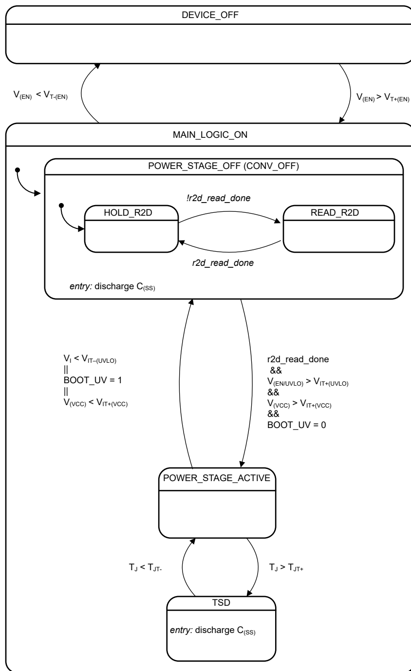
图 8-29. State Diagram
