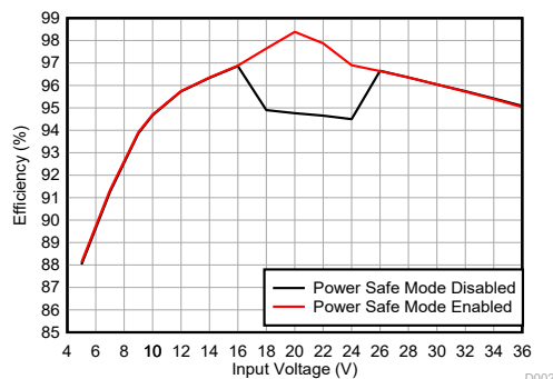
效率与输入电压间的关系, V_O = 20V , I_O = 5A
