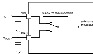
图 8-11. VMAX Supply Scenario 3
