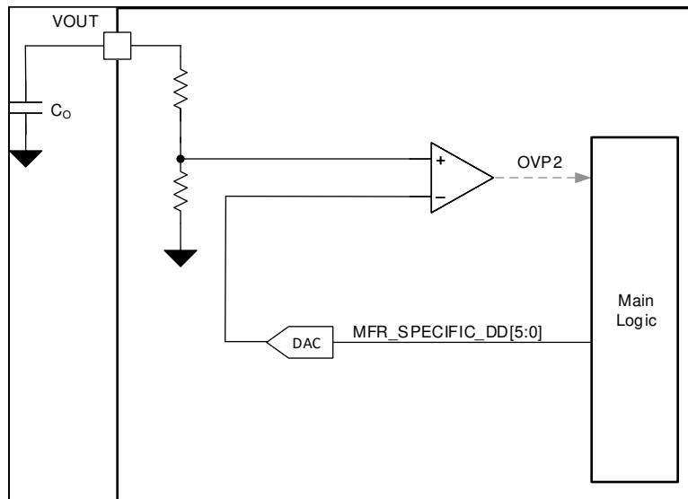
图 8-27. Functional Block Diagram OVP2
