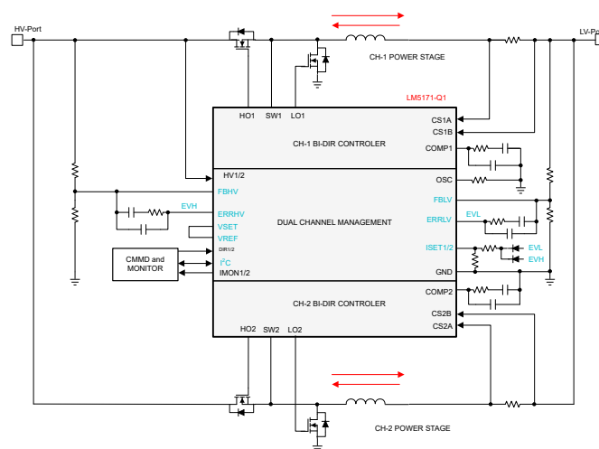
简化版应用电路
