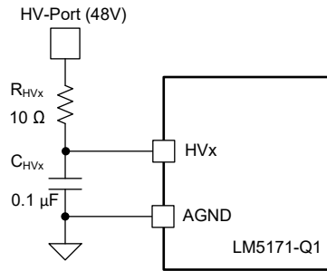
图 8-9. HVx Pin Configuration
