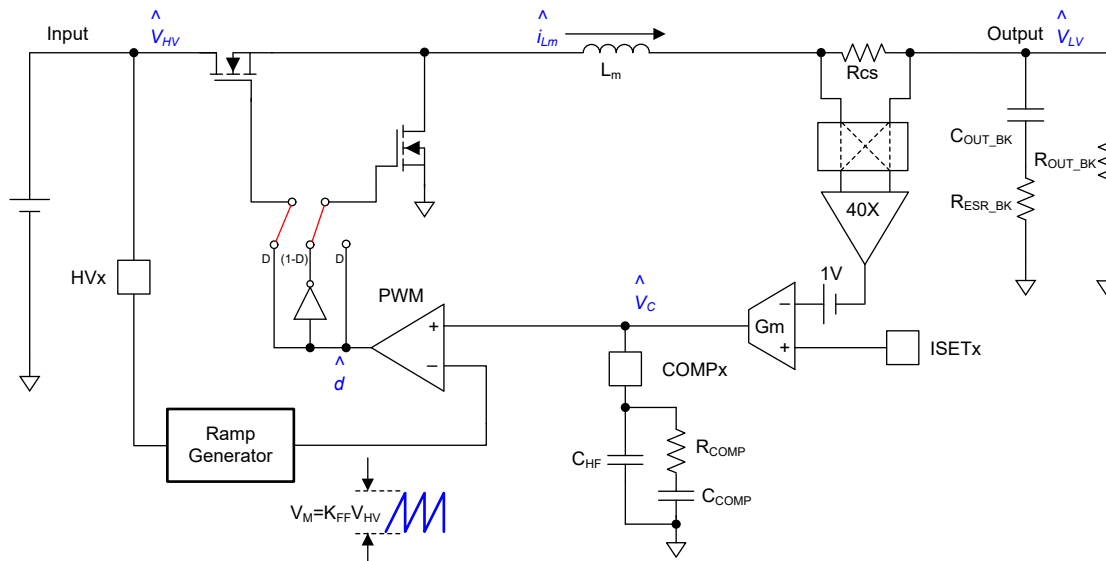
图 8-1. Buck Loop Block Diagram
