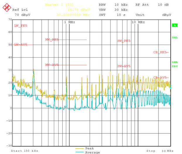
图 7-14. No-Load Switching
