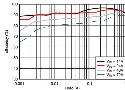
典型应用效率， V_{OUT} = 12V
