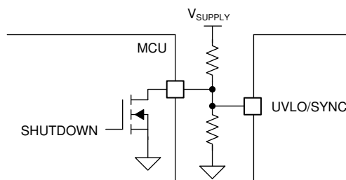
图 8-10. UVLO and Shutdown
