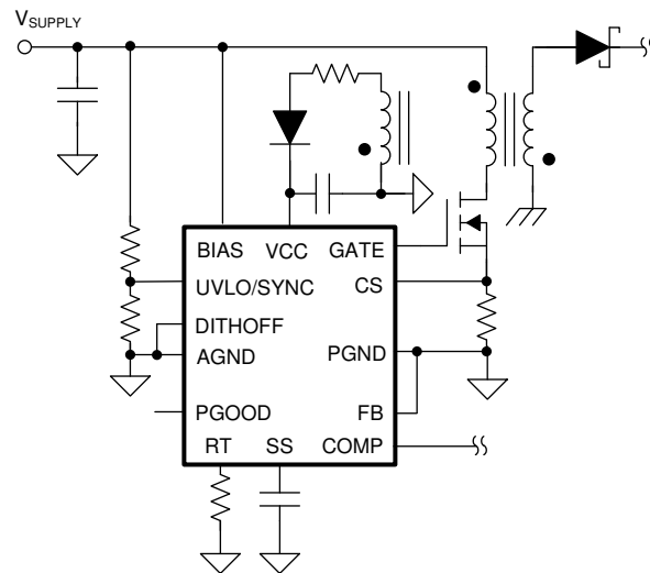
图 9-7. External VCC Supply (BIAS ≥ VCC)
