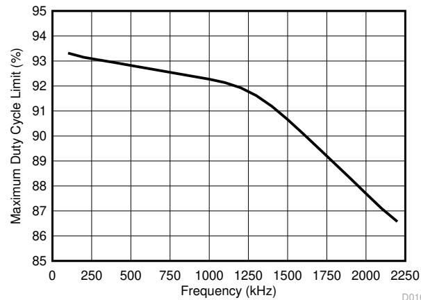
图 8-16. 最大占空比与频率间的关系
