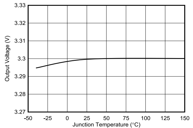
图 7-6. Fixed 3.3-V Output Voltage vs Temperature
