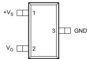
图 5-1. DBZ 封装 3 引脚 SOT-23 顶视图
