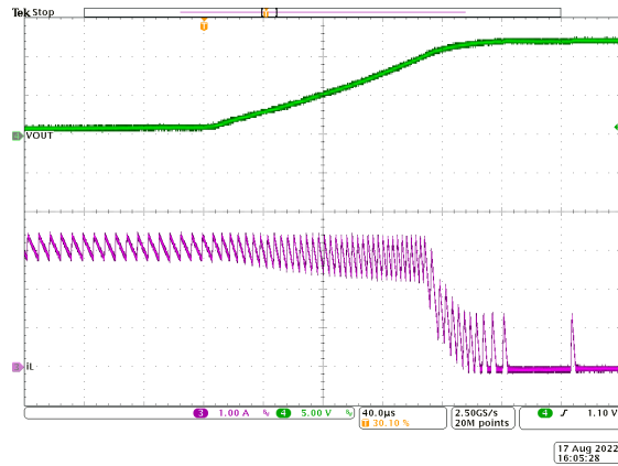
图 9-8. Short-Circuit Recovery
