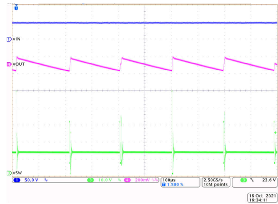
图 9-9. Light-Load Switching
