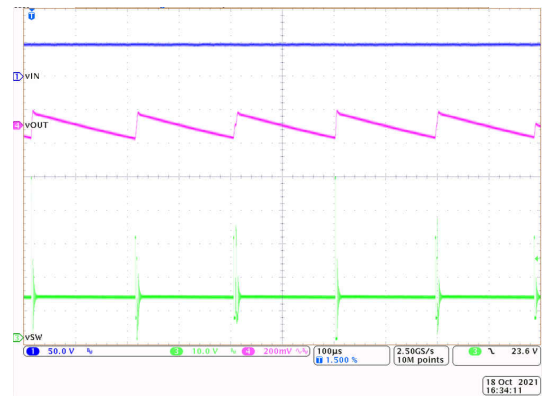
图 9-9. Light-Load Switching
