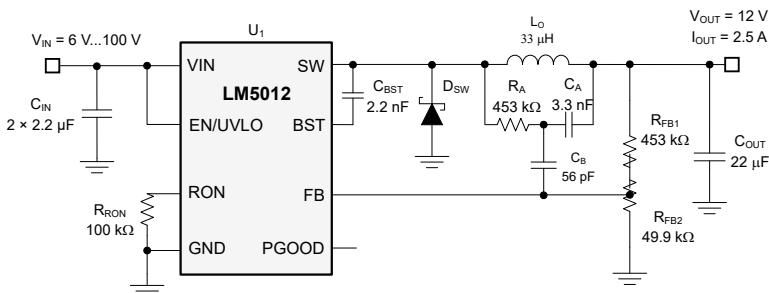
典型应用
