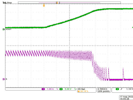
图 9-8. Short-Circuit Recovery
