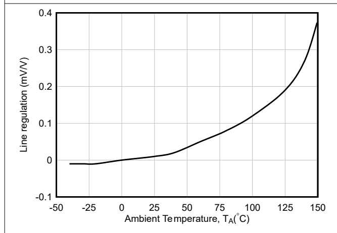
图 6-29. 线路调整与环境温度间的关系
