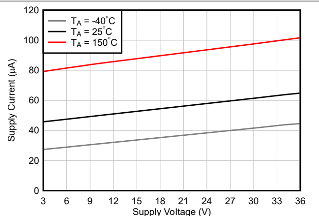
图 6-26. 电源电流与电源电压间的关系
