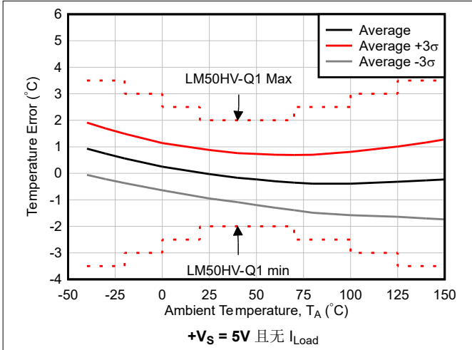
图 6-21. 精度与环境温度间的关系
