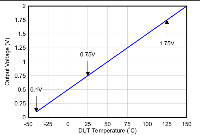
图 6-22. V_O 与环境温度间的关系
