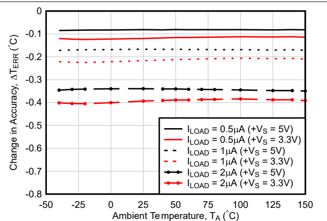
图 6-24. 精度与温度变化间的关系
