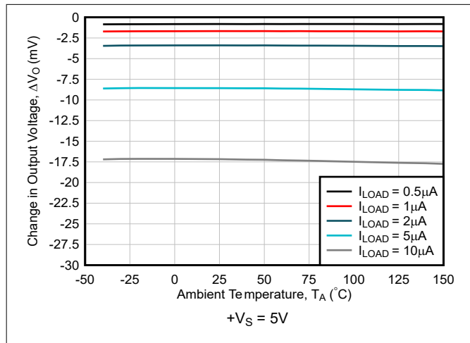
图 6-27. 负载调节与环境温度间的关系
