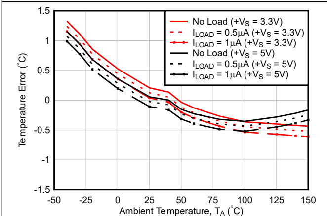
图 6-23. 不同负载下精度与环境温度间的关系
