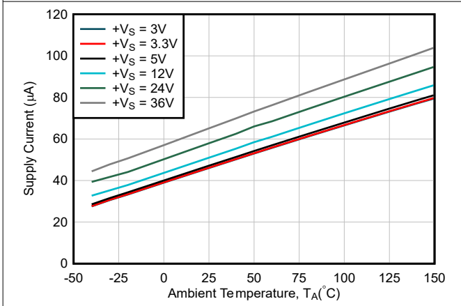
图 6-25. 电源电流与环境温度间的关系
