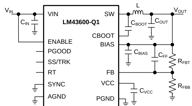
简化原理图
