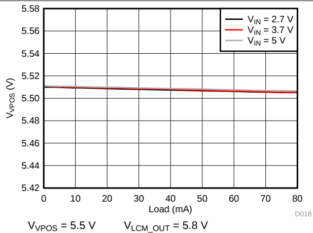
图 21. V_{VPOS} Load Regulation
