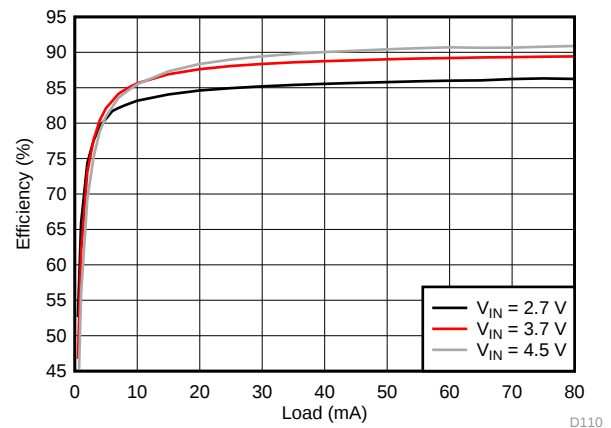
图 158. VPOS Efficiency
