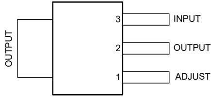
图 4-1. DCY 封装、3 引脚 SOT-223 (顶视图)
