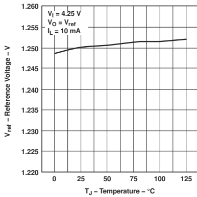
图 5-7. 温度稳定性与温度间的关系 (旧芯片)
