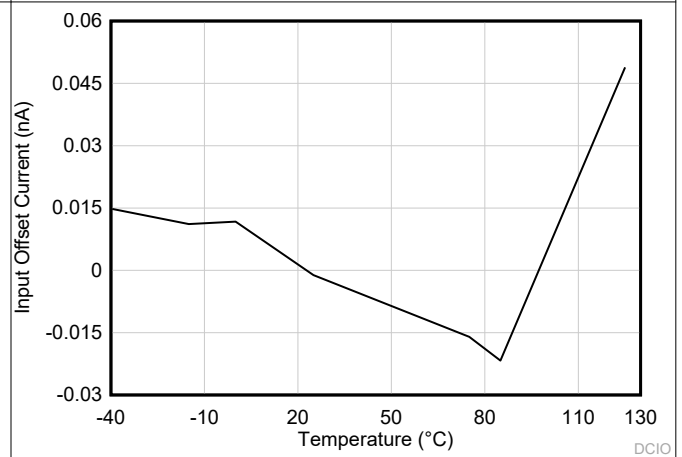
图 5-10. 输入失调电流与温度间的关系
