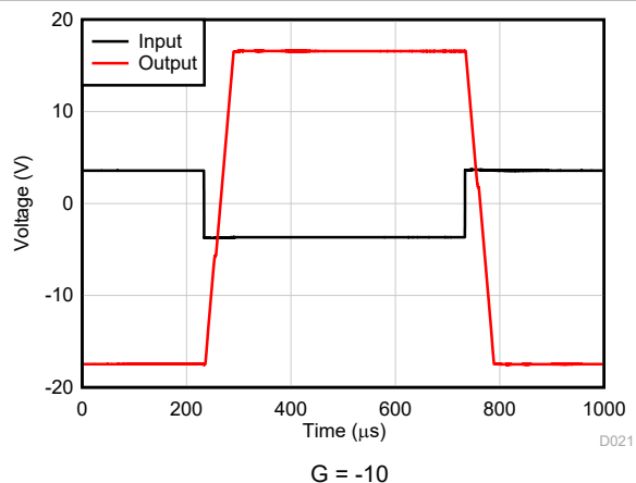
图 5-28. 过载恢复
